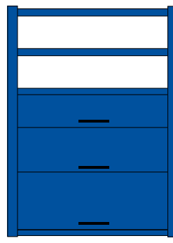
1 Fachboden 150 kg, 2 x Fachboden 500 kg, 1 x Schublade FH 250 mm, VA 500 kg, NH 120 mm, 1 x Schublade FH 350 mm, VA 500 kg, NH 220 mm, 1 x Schublade FH 450 mm, VA 500 kg, NH 320 mm, Sockelboden 50 mm
